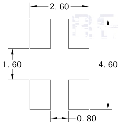
图 4 封装详细尺寸图
