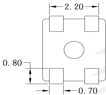
图 2 封装底面尺寸图
